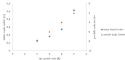
Gambar 12. Hubungan TSR, lebar sudu turbin, dan jumlah sudu turbin
