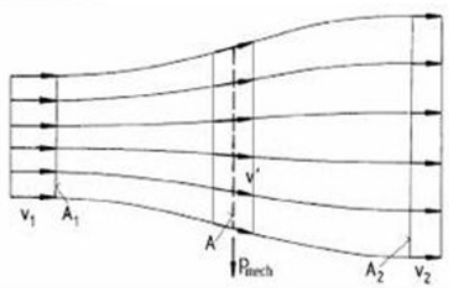
Gambar 5. Kecepatan angin melewati rotor (Gundtoft, 2009)
