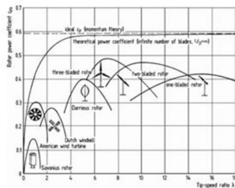
Gambar 6. Grafik perbandingan C_p dan TSR (John, 2012)
