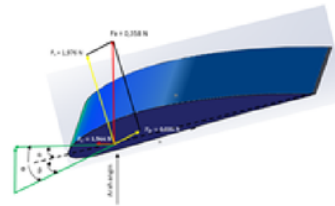
Gambar 9. Gaya-gaya pada sudu
