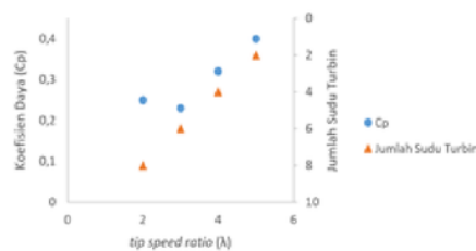
Gambar 10. Hubungan TSR, C_p , dan jumlah sudu turbin
